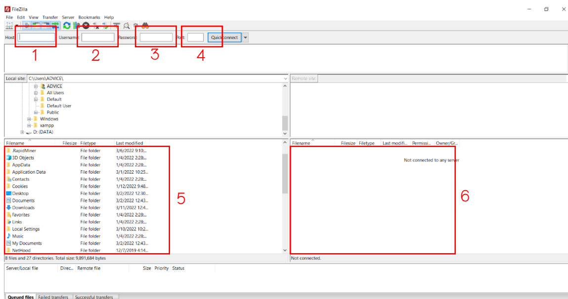
ภาพที่ ก.1 หน้าโปรแกรม FileZilla ใส่ข้อมูลชื่อและรหัส
